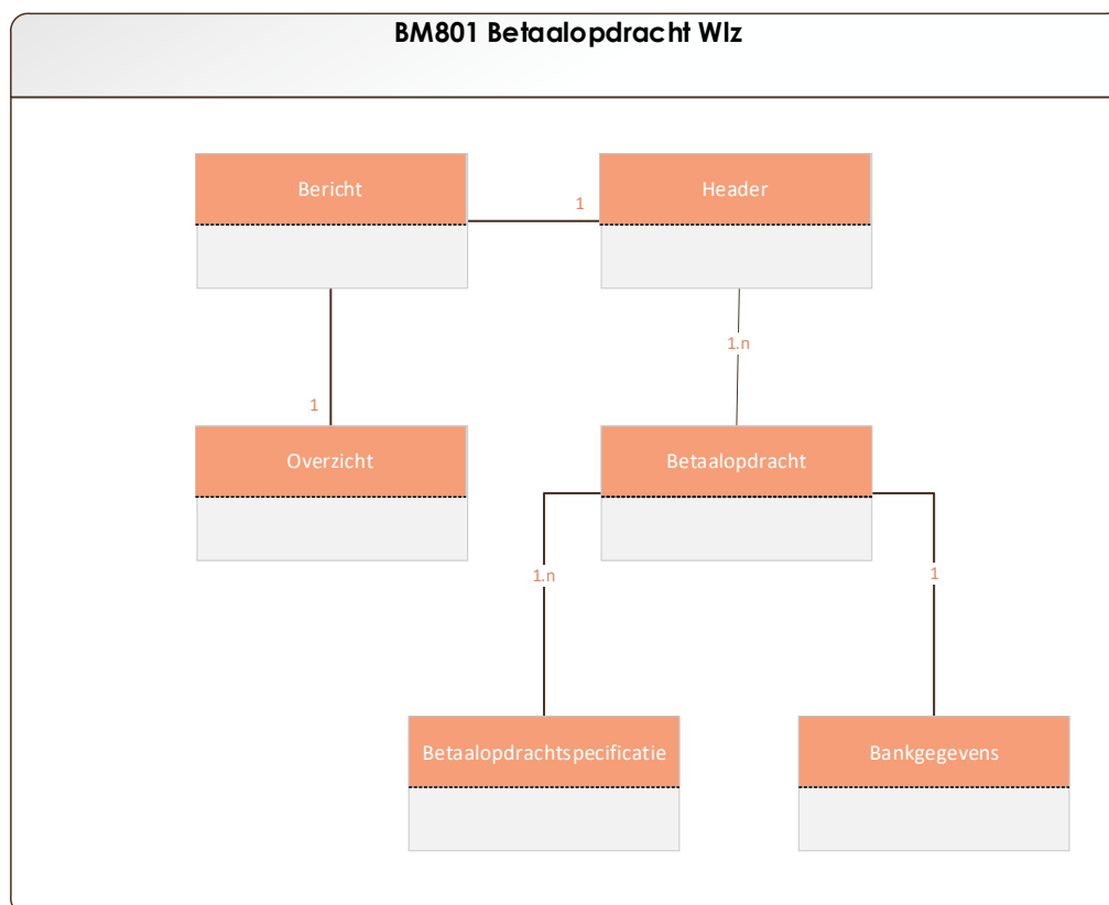
Figuur 1-1 Klassendiagram Betaalopdracht Wlz
