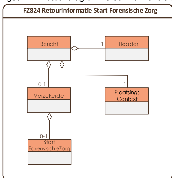
Figuur 1-1 Klassendiagram Retourinformatie Start Forensische Zorg
