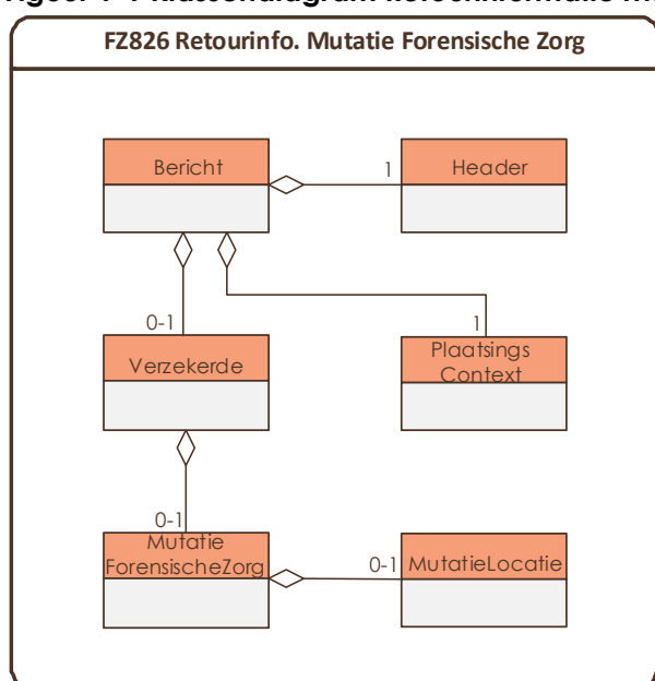
Figuur 1-1 Klassendiagramm Retourinformatie Mutatie Forensische Zorg
