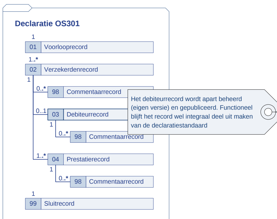
Figuur 5-1 Logische bestandstructuur OS301
