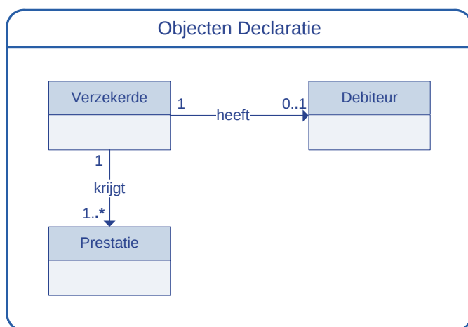
Figuur 4-1 Objectmodel Declaratie zorg overige sectoren
